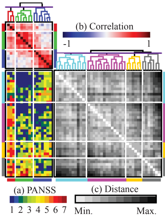
◀圖六 以樹狀結構將資料作適當的分群
