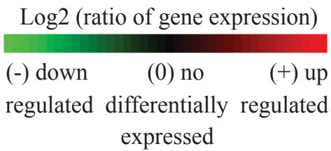
圖二 微陣列基因表現之雙向性色譜
