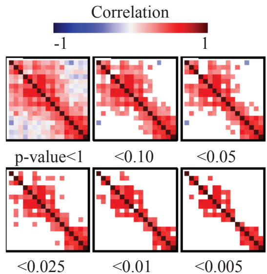
►圖九 分段式(sectional)全矩陣視覺化
