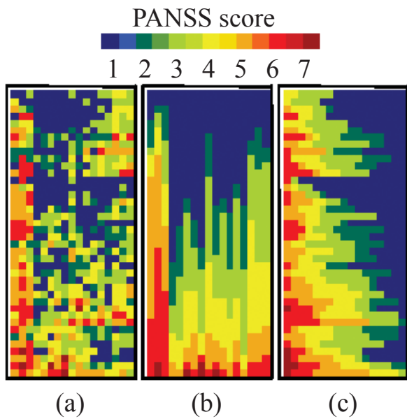
▲圖八 全矩陣視覺化之沈澱圖
