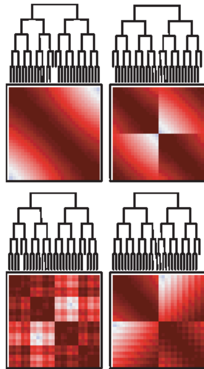
圖五 不同節點翻轉機制在同一個樹狀結構與關係矩陣上造成的排序差異
