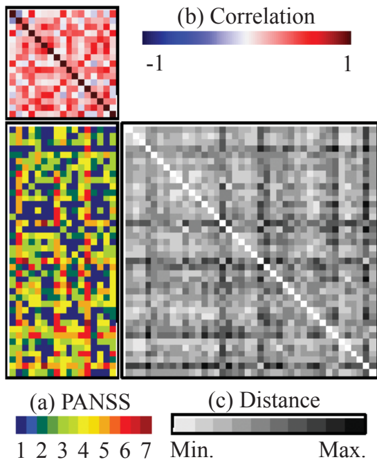
圖一 原始資料與關係矩陣之呈現
