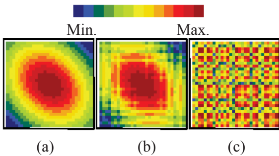
圖三 Robinson 與準-Robinson 矩陣
