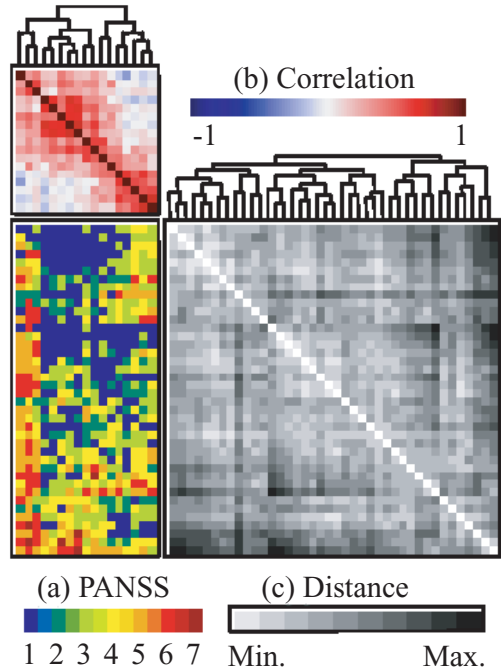
圖四 排序後之關係矩陣與資料矩陣
